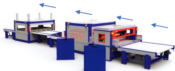
Ligne complete de fabrication
